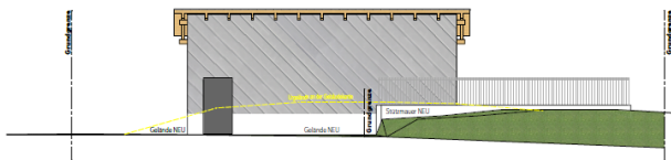
Ansicht: Süd
