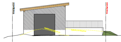
Ansicht: West
